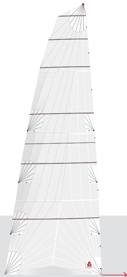
MODÈLE À CORNE DÉCONNECTABLE EN COUPE TRIRADIALE
