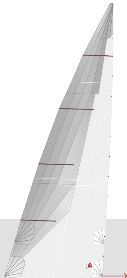
MODÈLE EN COUPE TRIRADIALE
